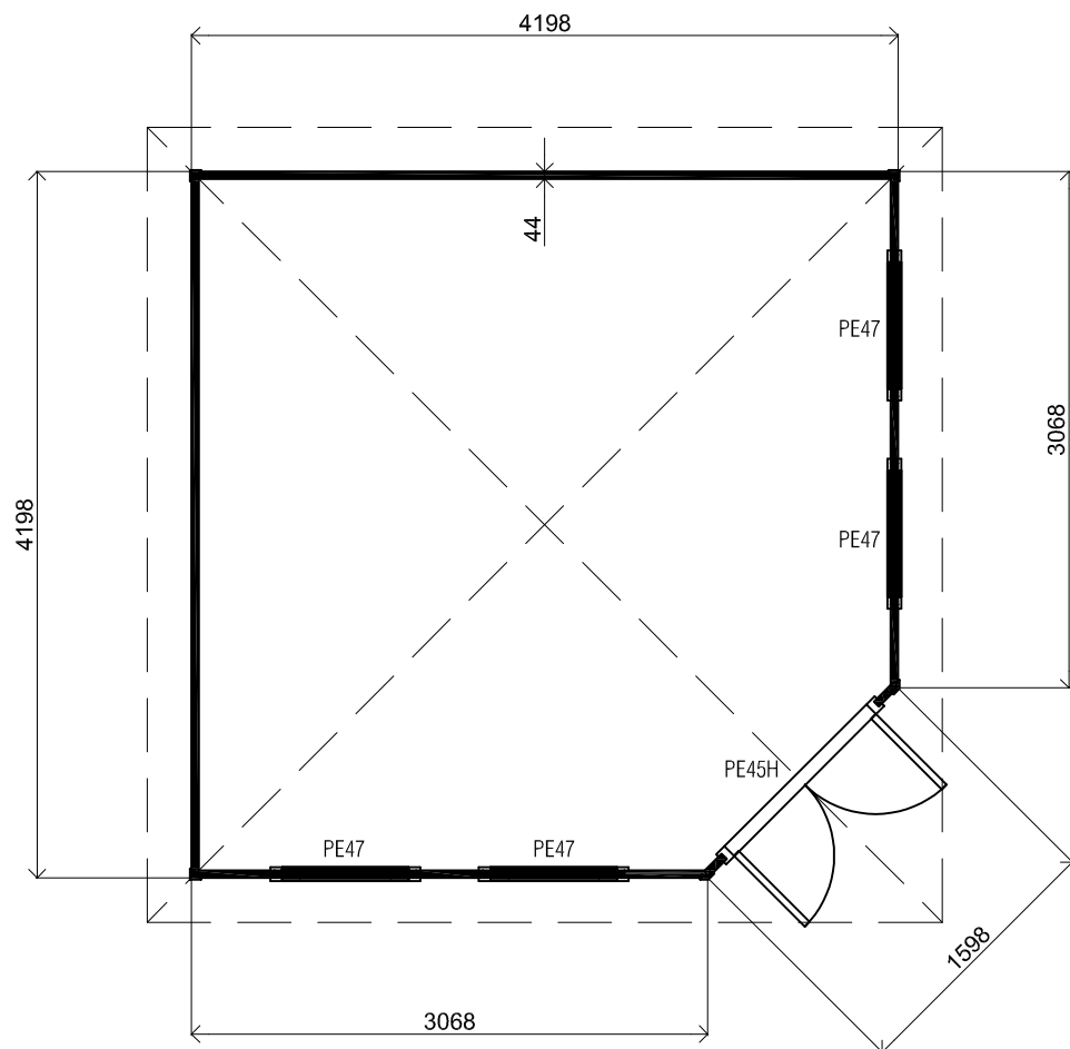
Plattegrond / Plan
